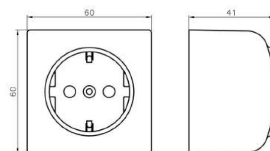
Gniazdo pojedyncze z uziemieniem schuko
