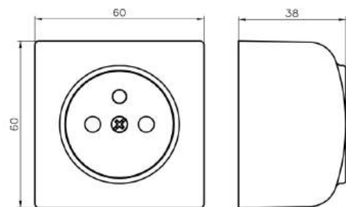
Gniazdo pojedyncze z uziemieniem
