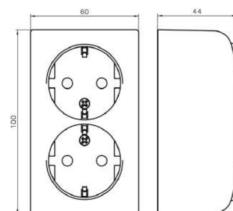
Gniazdo podwójne z uziemieniem schuko
