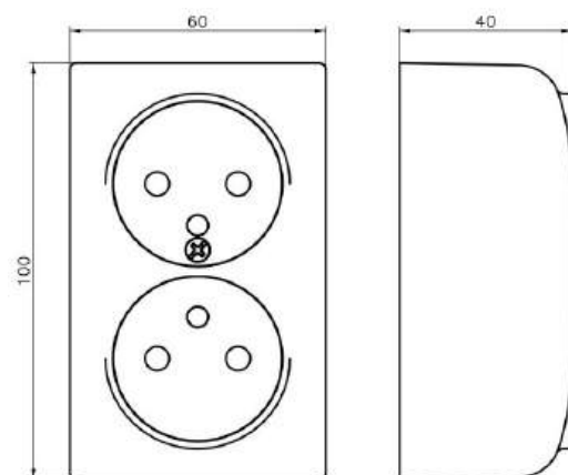
Gniazdo podwójne z uziemieniem
